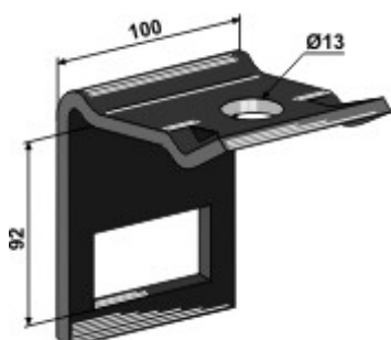
Bride pour tube 80x80
